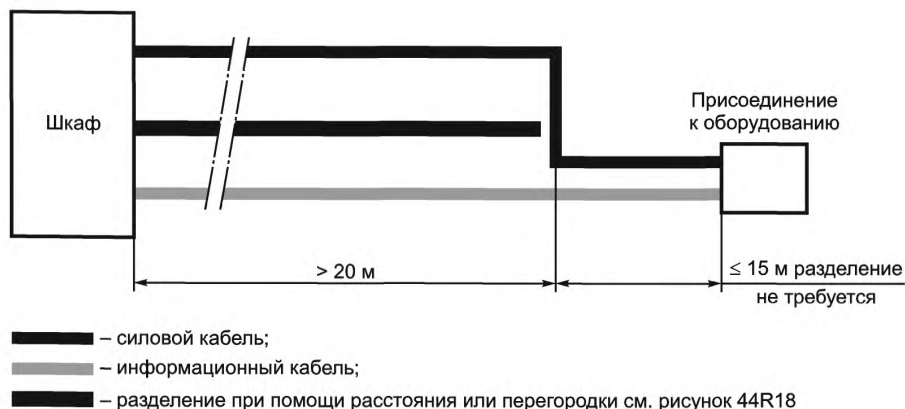
Рисунок 44.R17В — Разделение силовых и информационных кабелей при длинах кабельной трассы > 35 м
