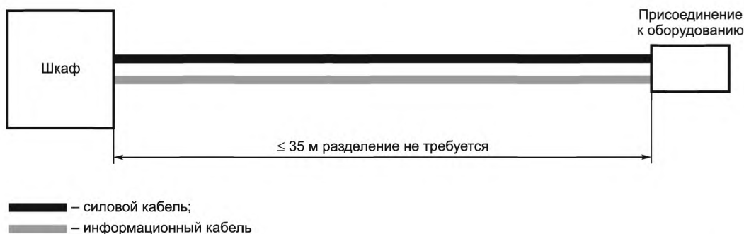
Рисунок 44.R17A — Разделение силовых кабелей и кабелей информационных технологий при длинах кабельной трассы ≤ 35 м
