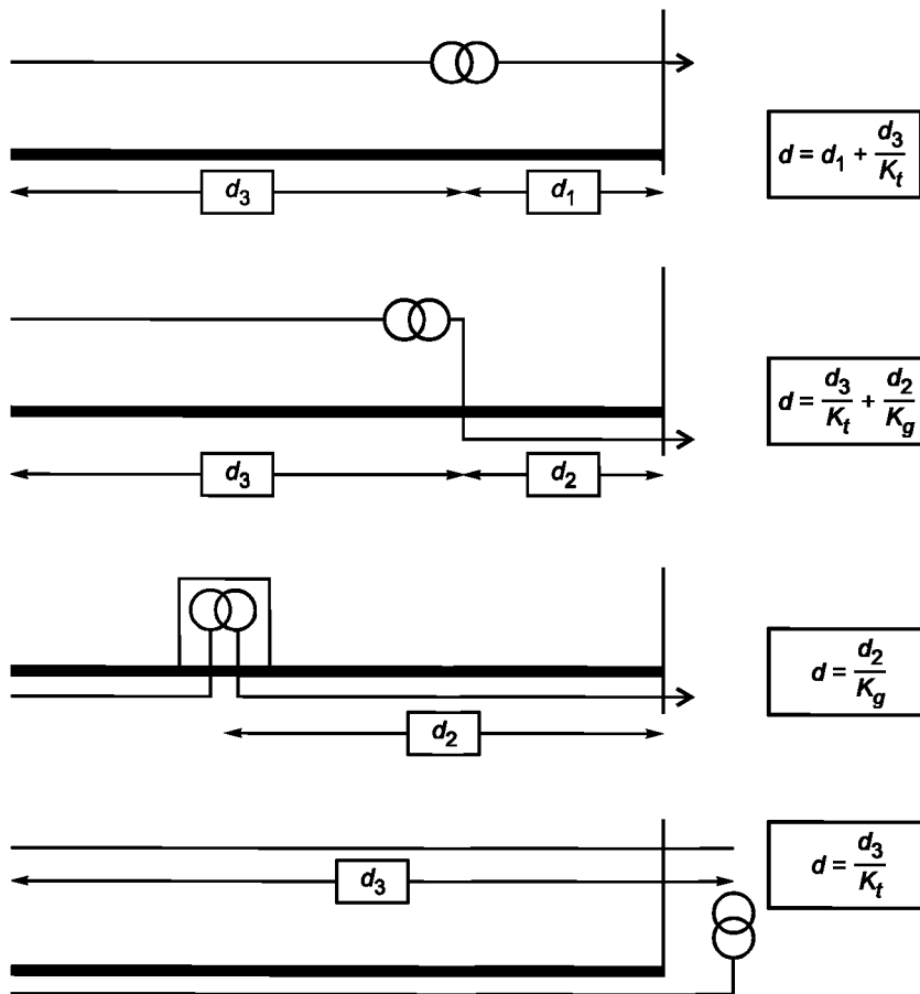
Рисунок 44.Q — Примеры использования d_1 , d_2 , и d_3 для определения d
